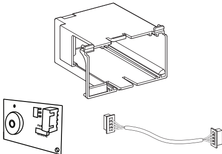
Fig. 84 ATC 100 Kit P/N: 105708
